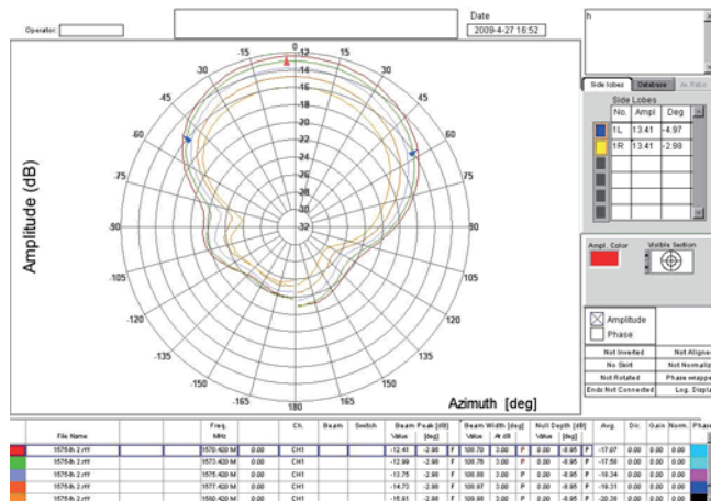
天线辐射方向图
