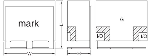
Dimension (尺寸) ( Unit:mm )
